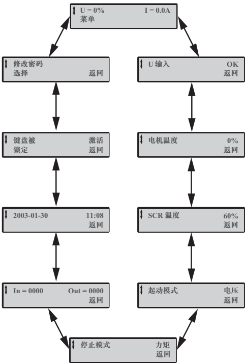
图1：主菜单显示
