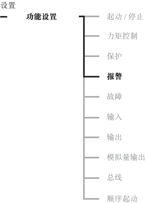
图 29：报警群组
