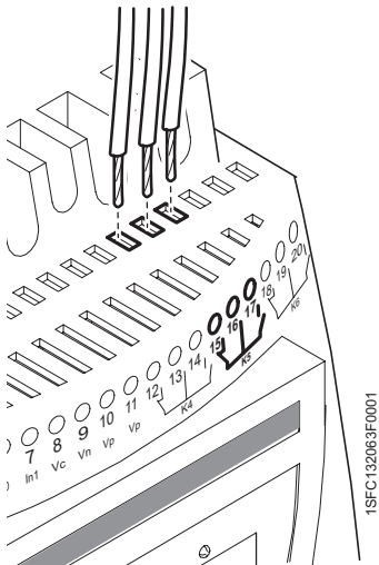
图 25：端子 15、16、17
