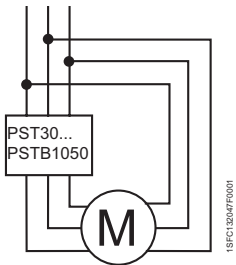
图2：内接
