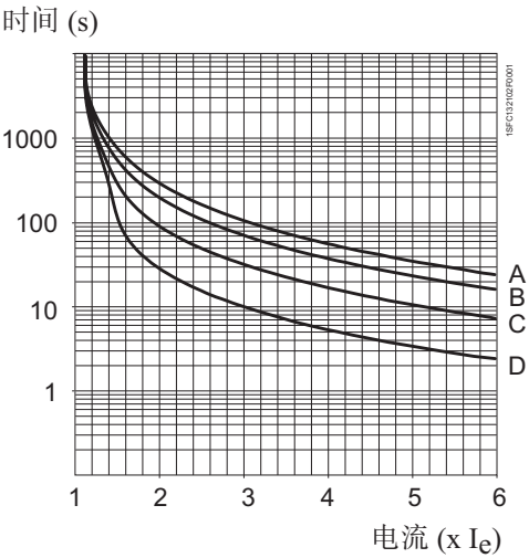
图 13：电子过载的脱扣曲线
