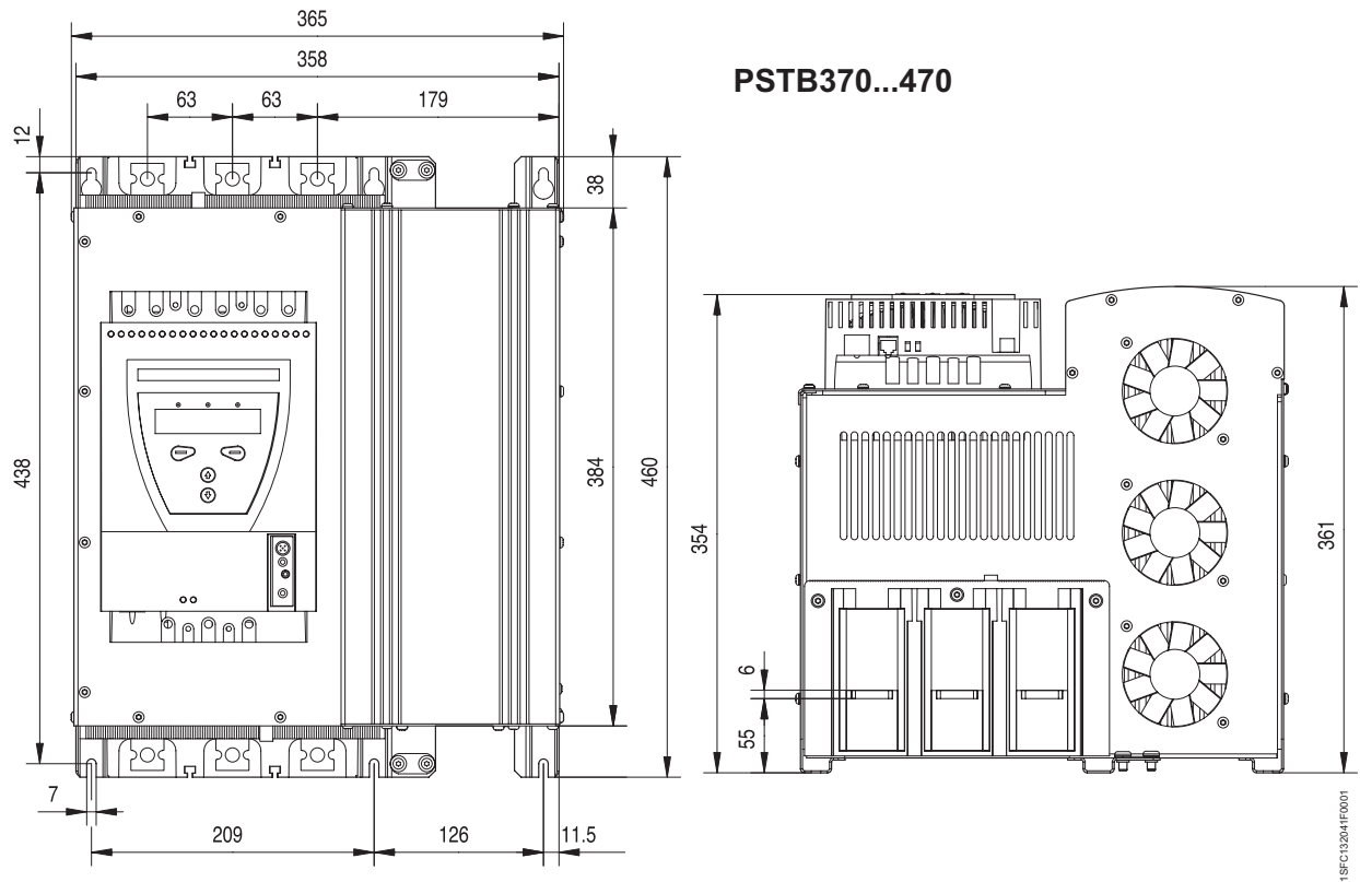
图6：PSTB370 ... 470 的尺寸图 (mm) (1mm=0.0394 吋)
