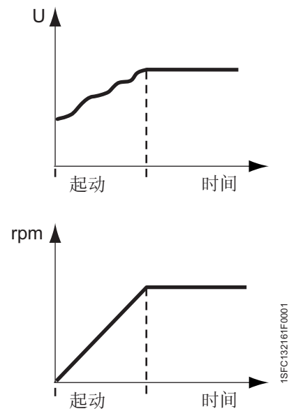
图2：力矩斜坡
