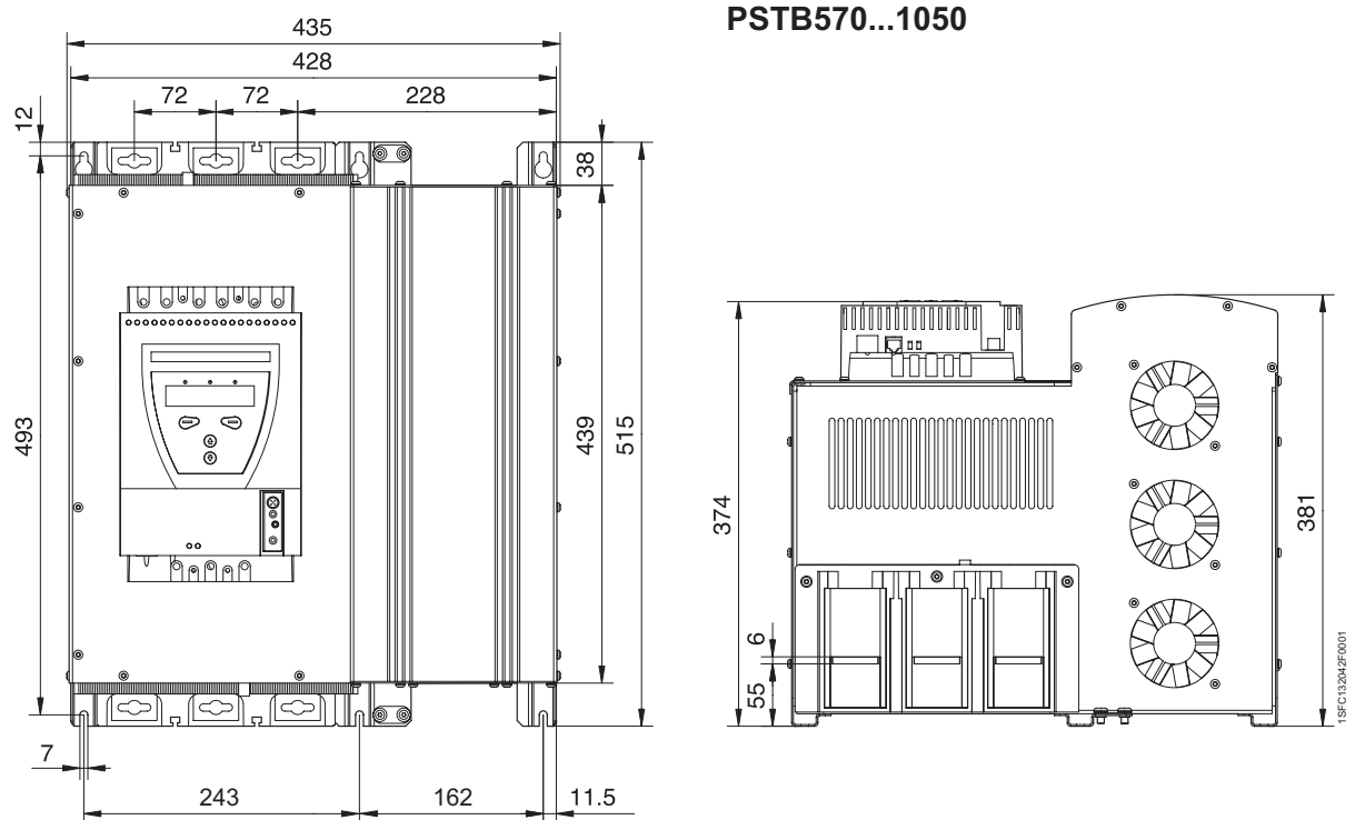
图7：PSTB570 ... 1050 的尺寸图 (mm) (1mm=0.0394 吋)
