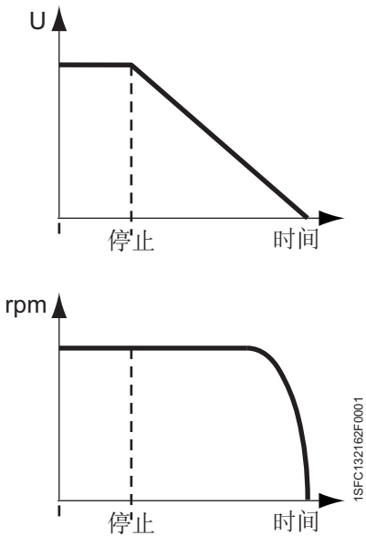
图 3：电压斜坡
