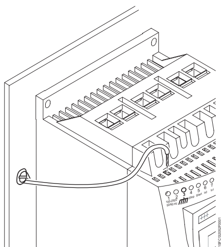
图 8：功能接地
