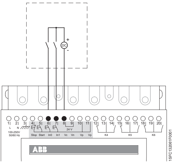
图 15：外部控制电压
