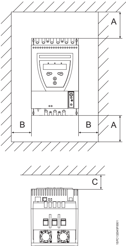
图3：与墙/前面板的最小距离
