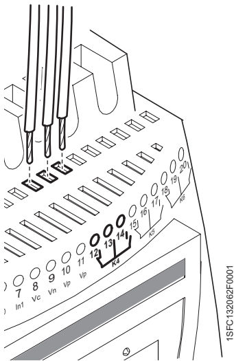
图 24：端子 12、13、14
