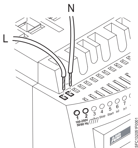
图 7：控制回路电源
